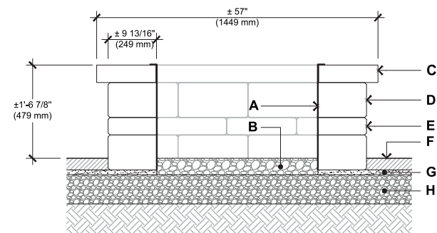
COUPE 1-1
