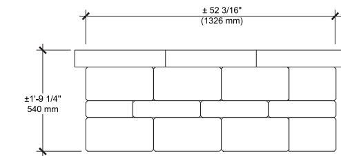
ÉLÉVATION A
